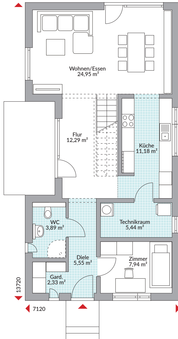
Erdgeschoss 73,57 m 2
